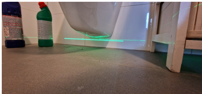
Manglende dreneringsløsning for innebygget sistene.
