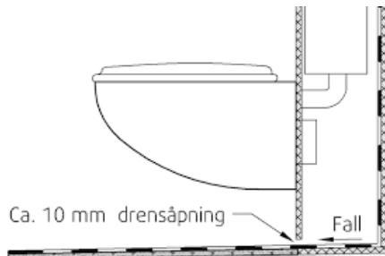
Normal montering av innbygget klosettsisterner.
