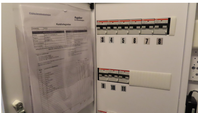
Sikringsskap.
