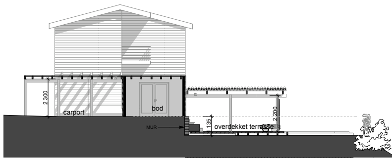
Snitt AA
