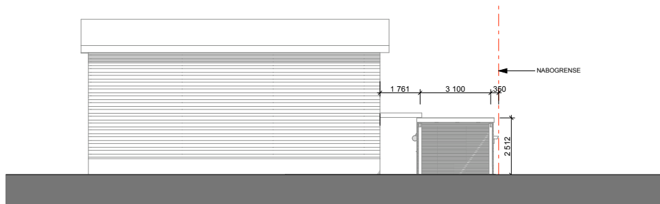
Fasade sør
