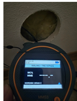
Måling av trefukt i lukket veggkonstruksjon mellom stue og dusjsone.
