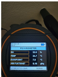
Måling av relativ luftfuktighet i lukket veggkonstruksjon mellom stue og dusjsone.
