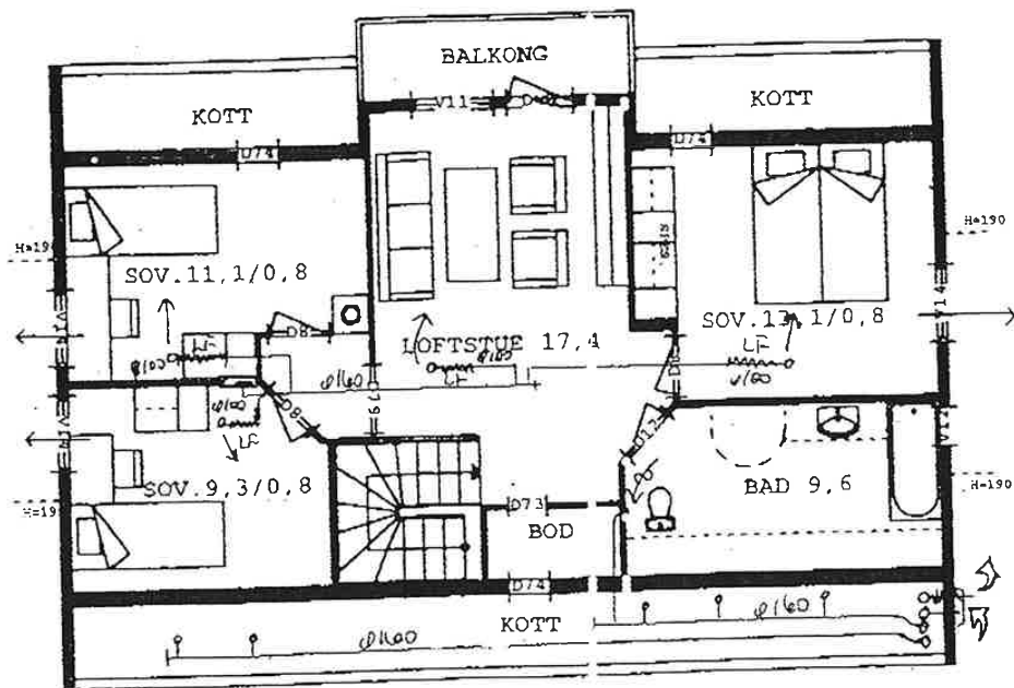
PLAN 2. ETASJE
