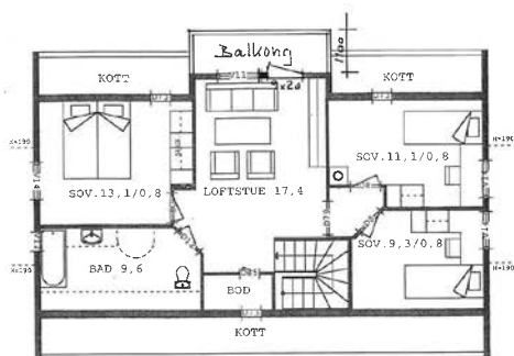
PLAN 2. ETASJE
