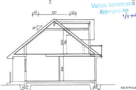
HOVEDSNITT
