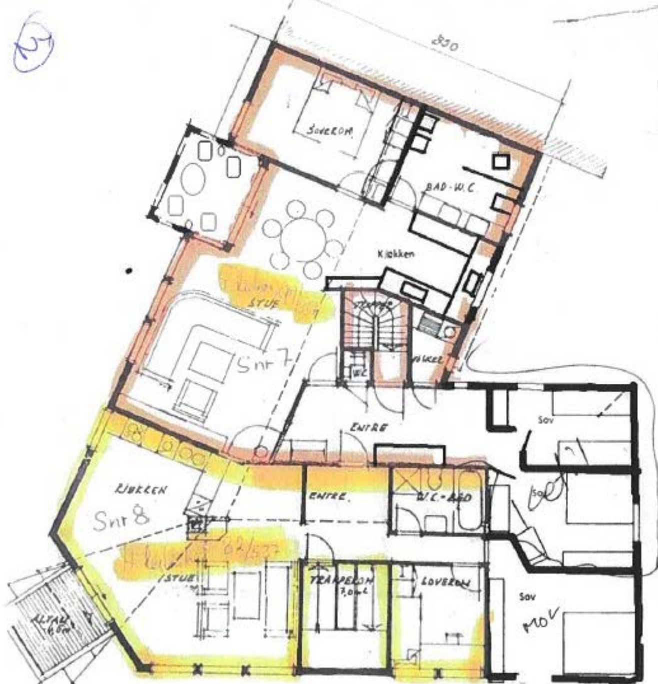
Plan 3. etasje (loft.).
