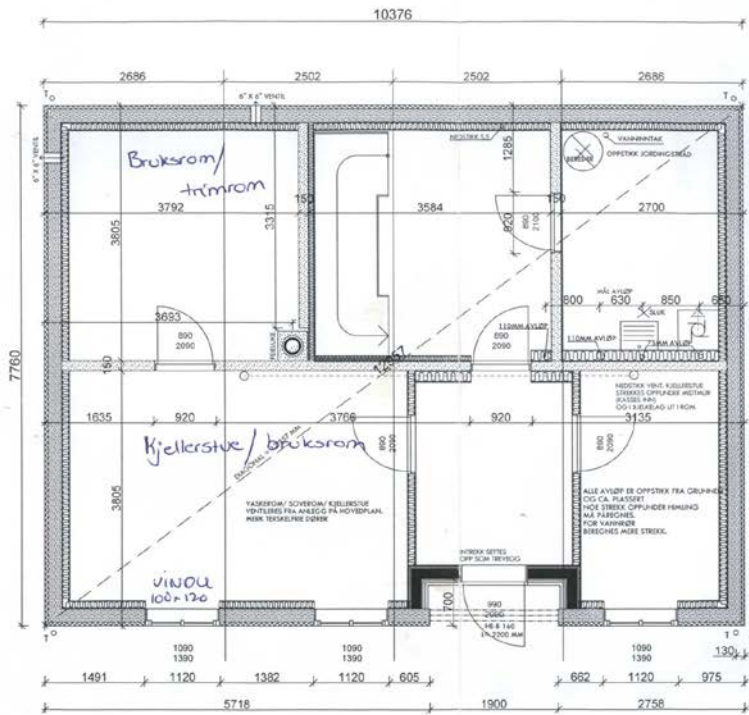
SOKKELPLAN MÅLESTOKK 1:50
