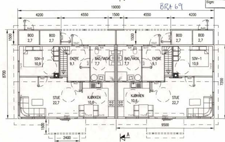
HOVEDPLAN
