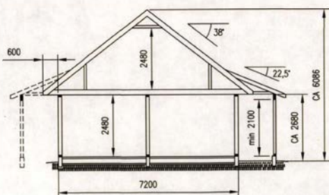
SNITT A-A
