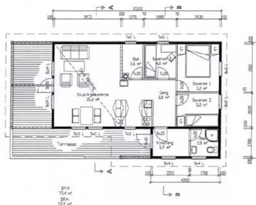
PLAN 1. ETASJE
