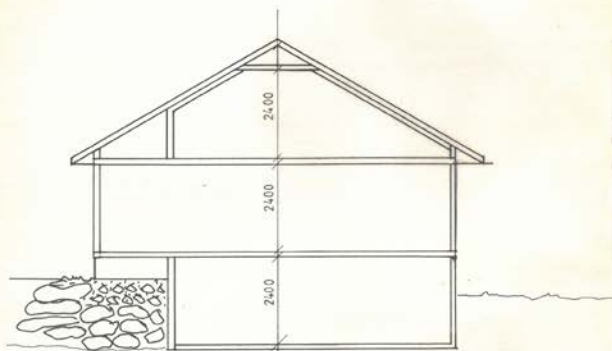
SNITT NYBYGG
