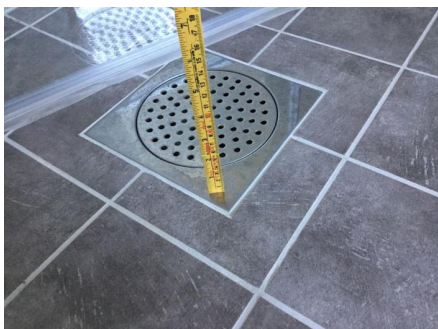
Fall til sluk er kun 8 mm.
