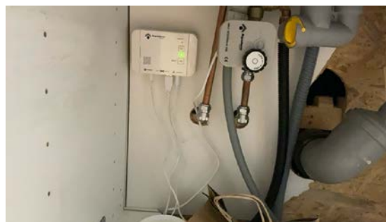
Vannstoppsystem.
