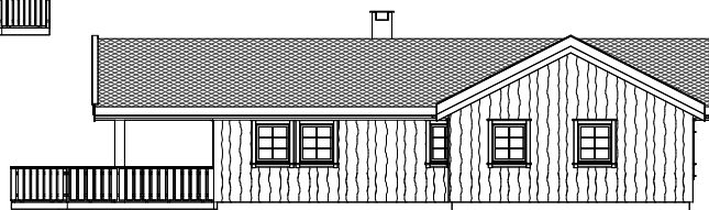
Fasade 2 1 : 100
