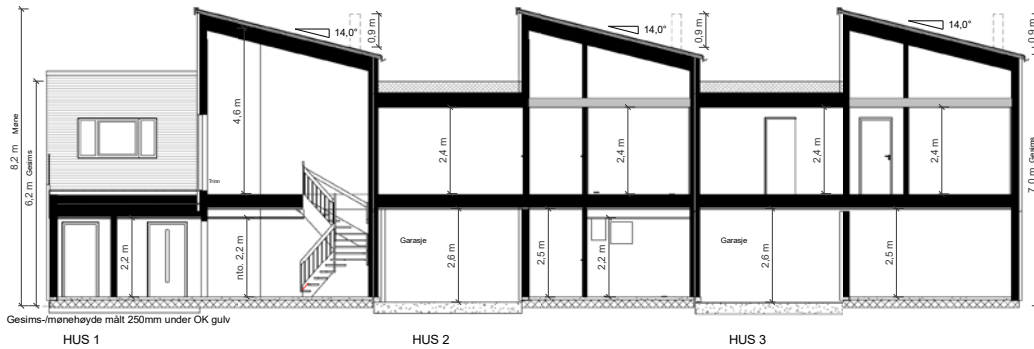
Snitt A
