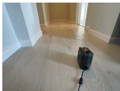
Nivellering stue/kjøkken og entré, avvik ca. 10-20 mm
