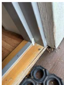
Utett mellom dørblad og dørkarm nede. Forsøkt utbedret med liten pakning. Tetter ikke tilstrekkelig når døren er lukket.
