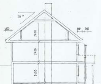
SNITT
