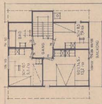
plan 2 etasje
