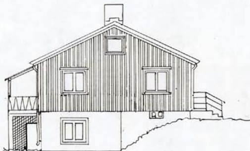
FASADE SYD / VEST
