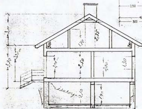
SNITT
