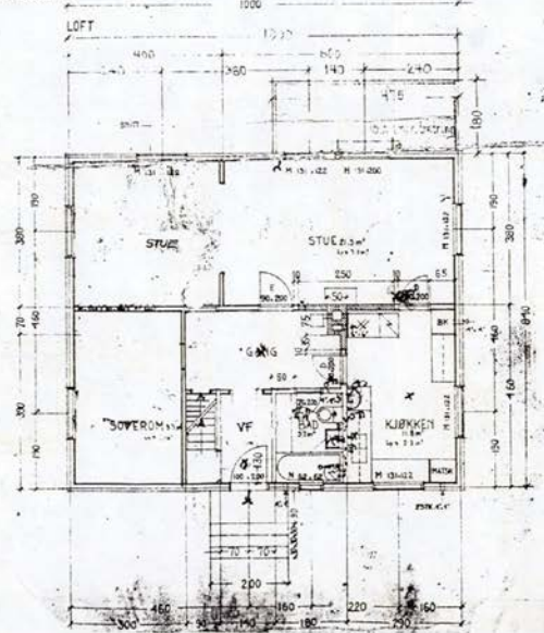
PLAN 1.ETASJE
