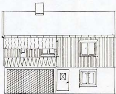
FASADE NORD / VEST
