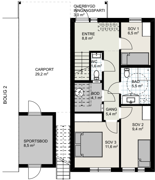
1. Etasje
