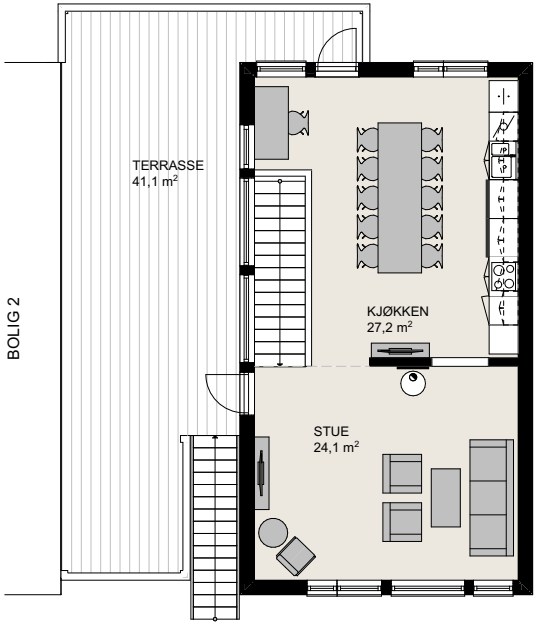
2. Etasje
