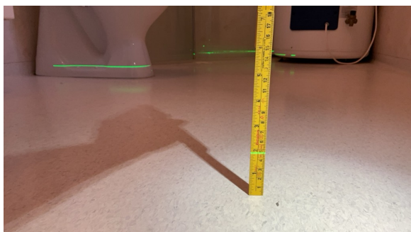
Lokalt motfall mot dør ved at høyeste punkt er midt i rommet.
