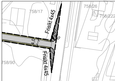
Dimensjoner, kryss/avkjørsel 1:750
