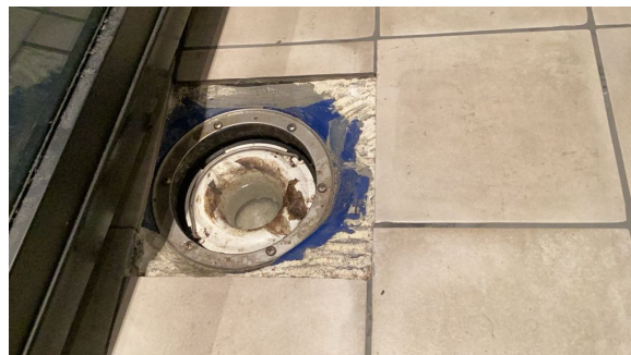
Synlig mansjett og membran, ingen slukrist.
