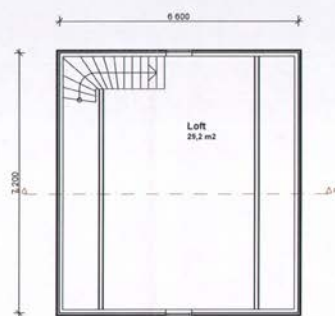
PLAN 1. ETG.
