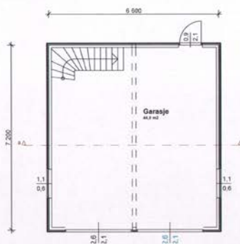
LOFTSPLAN
