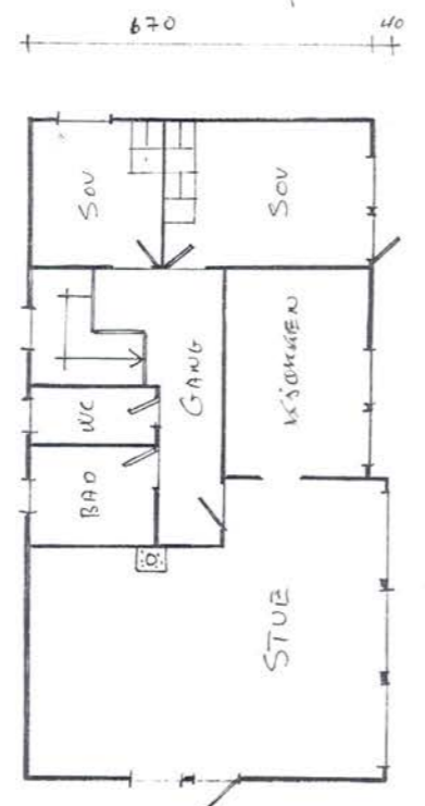
1. ETASJE FØR UTVIDELSE
