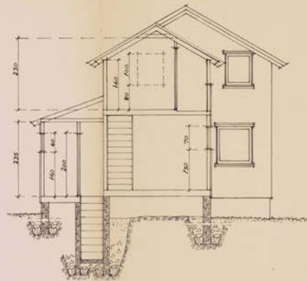
SNITT A-A.
