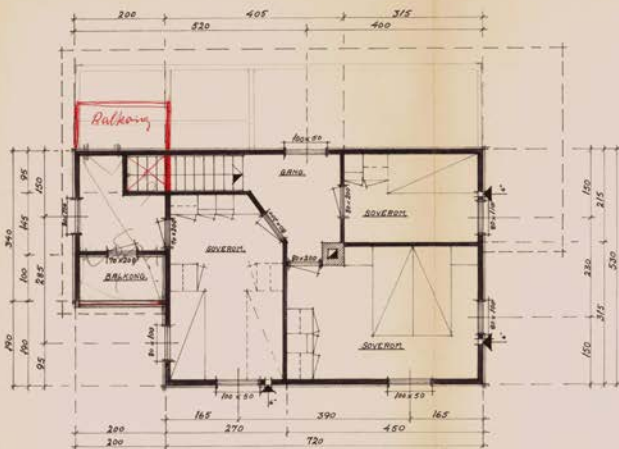
PLAN AV 2. ETASJE.
