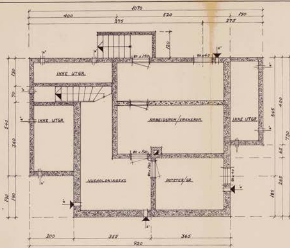
KJELLERPLAN.
