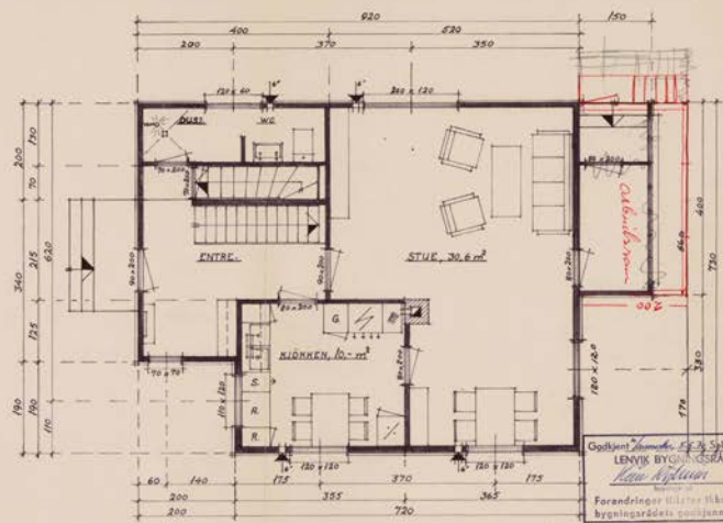
PLAN AV 1. ETASJE
