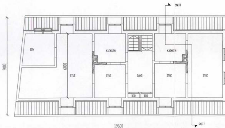
PLAN 2. ETASJE
