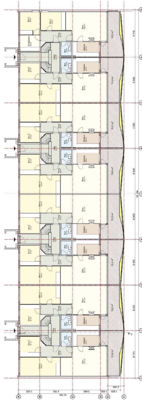
1:200
