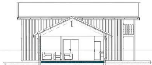
Snitt A5 1:100
