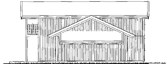
Fasade Øst 1:100
