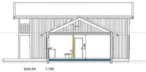
Snitt A4 1:100
