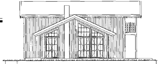
Fasade Vest 1:100
