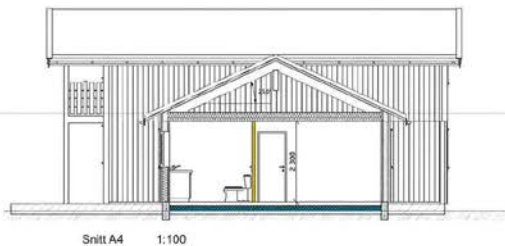
Snitt A4 1:100
