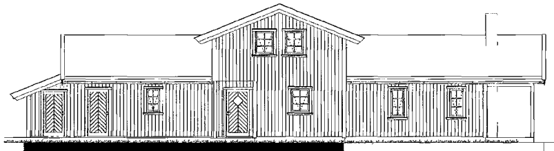
Fasade Nord 1:100
