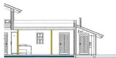
Snitt B3 1:100
