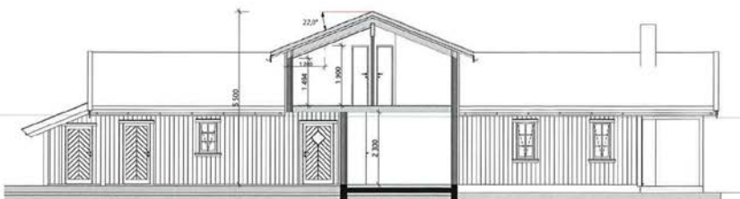
Snitt B2 1:100
