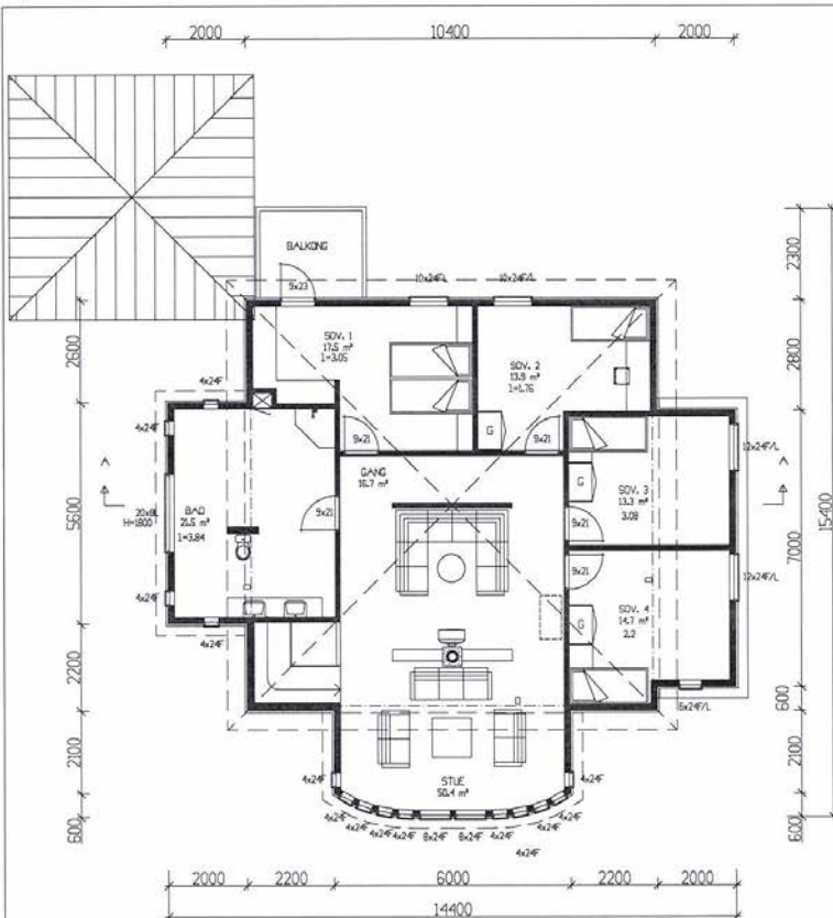
2. ETASJE
