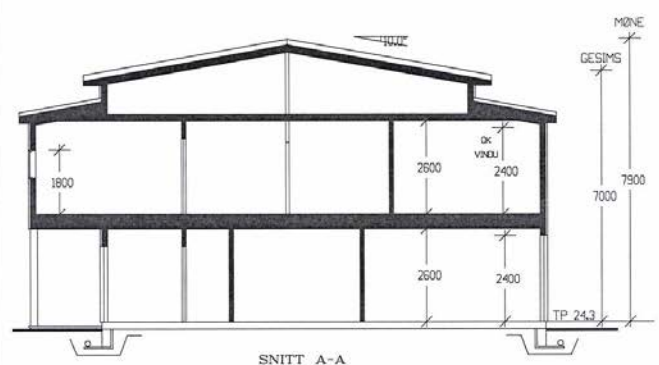
SNITT A-A
