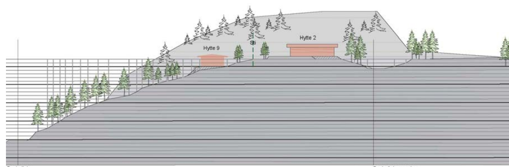
Snitt B - B
