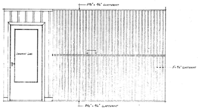
OPDRIS AV GITTERVEGG MOT TRAPP M/DØR IHNEN I STUE
