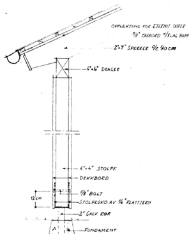
SØYLE VED HØVEDINNGANG MÅL 1:10
