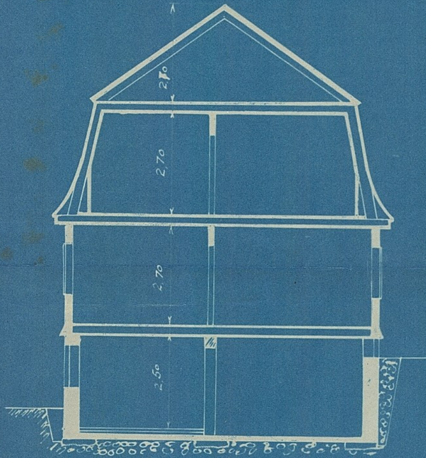
TVERSNIT
