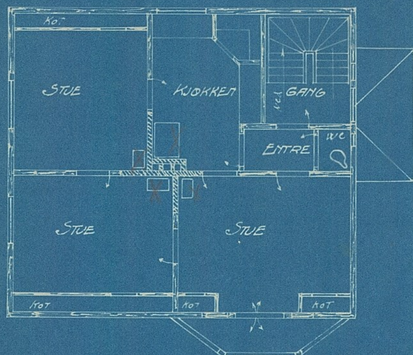
ANDEN ETAGE
