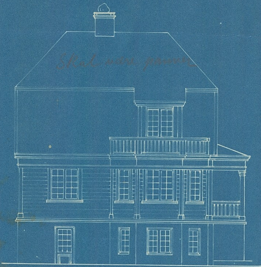
MOT ØST
