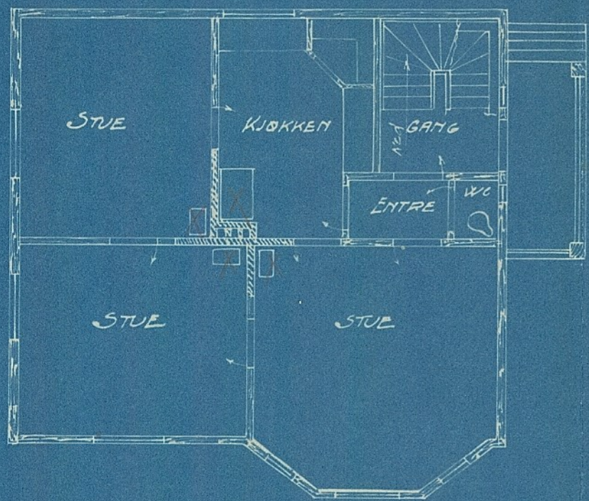
FØRSTE ETAGE
