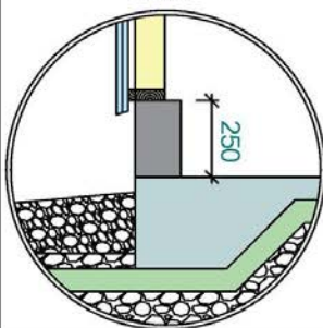
Snitt A
