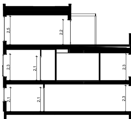
Snitt B
