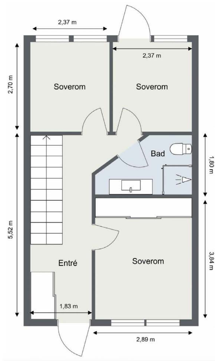
Rekkehus Etasje 1
