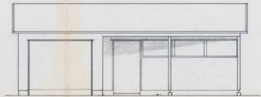
FASADE SØD
