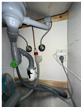
Røropplegg i kjøkkenbenk med Waterguard
