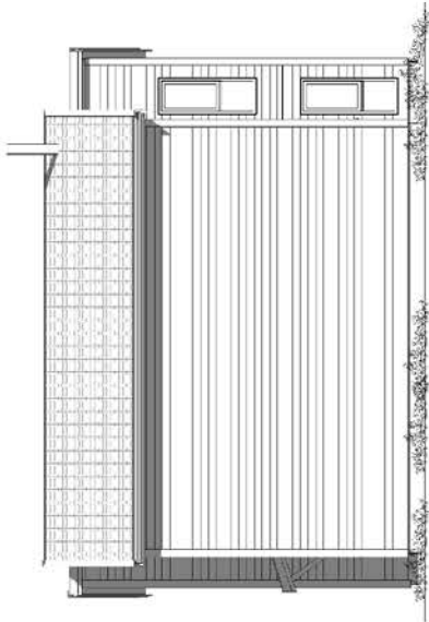
Fasade nord-øst 1 : 100
