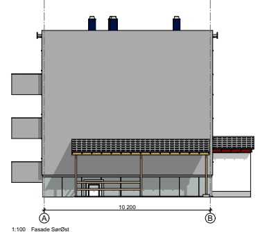
1:100 Fasade SørØst
