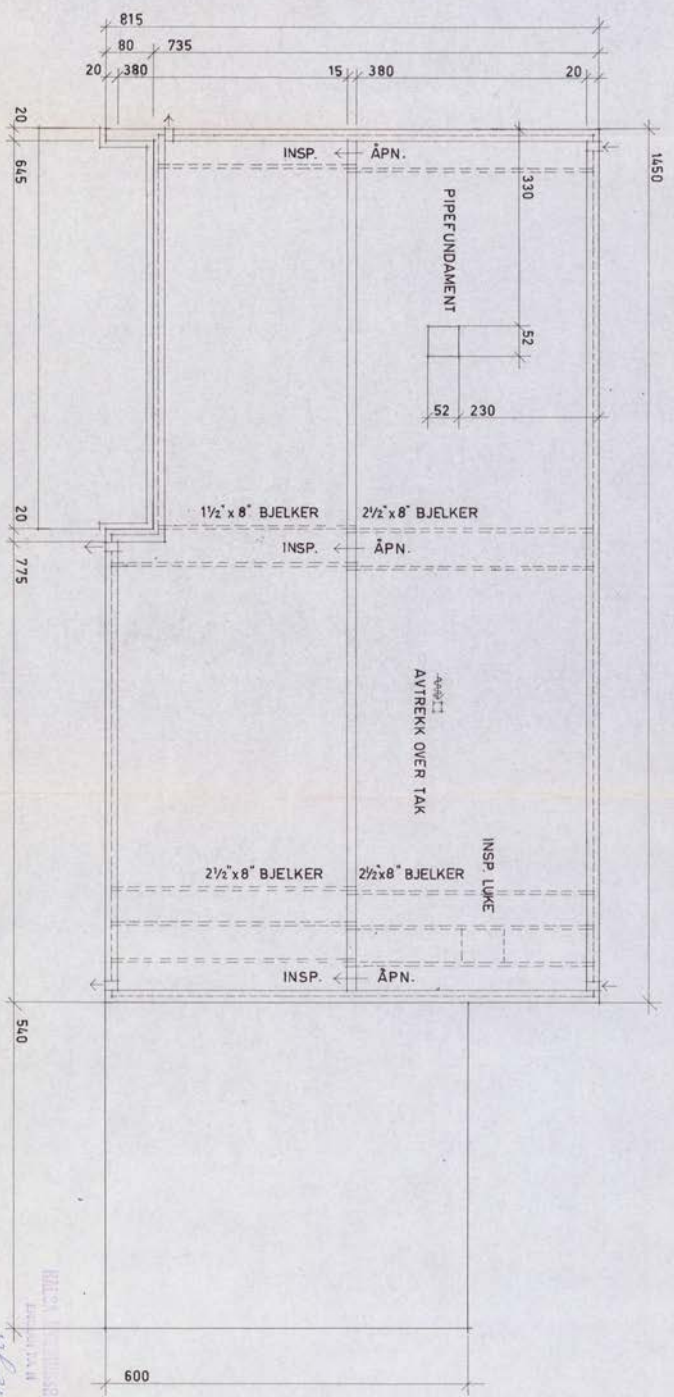
TEGN. NR. 3 FUNDAMENTPLAN MÅL 1:50 HUSBANKENS ARKITEKTKONTOR OSLO 8. 8. 67
