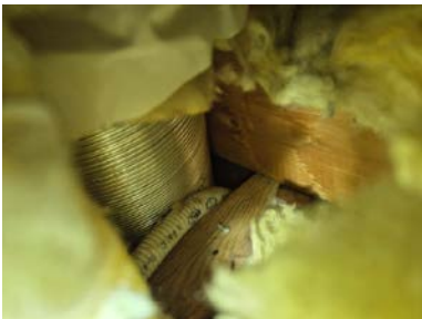
Brudd på dampspærre rundt rørgjennomføring.
