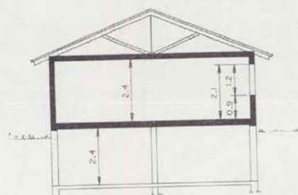
SNITT
