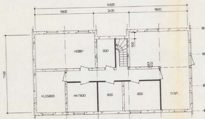
MIDLERTIDIG FUNDAMENTPLAN
