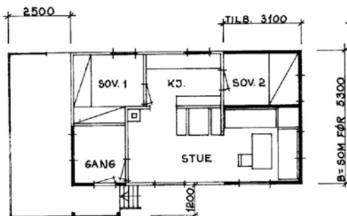
PLAN ETTER OMB/TILB. 1:100
