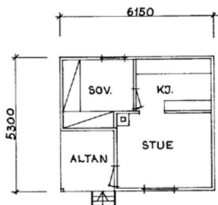
PLAN FØR OMB/TILB. 1:100
