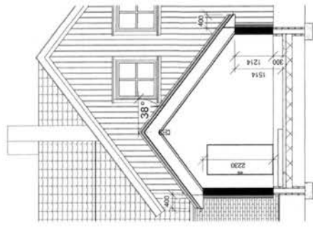
Snitt D 1 : 100
