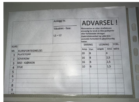
Kursoversikt i sikringskapp
