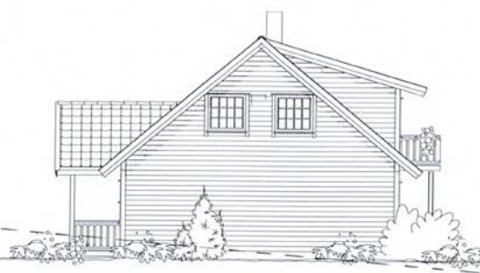
Fasade mot nordvest 1:100
