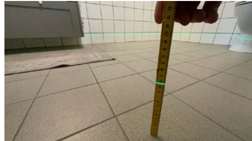
Målt gulvrområde med motfall ved yttervegg siden av dør.
